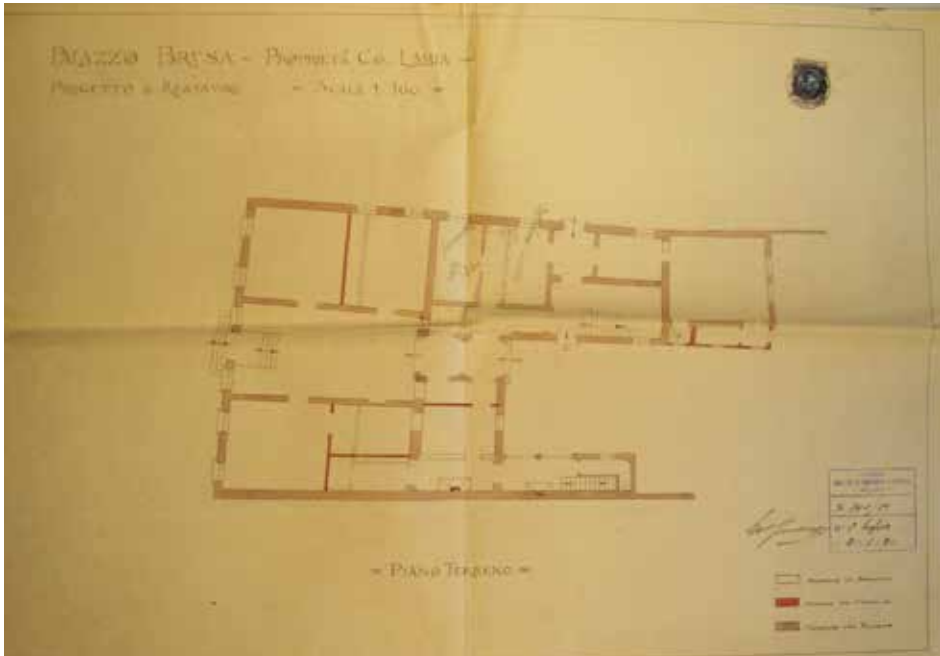
Figura 1. Pianta del piano terreno
