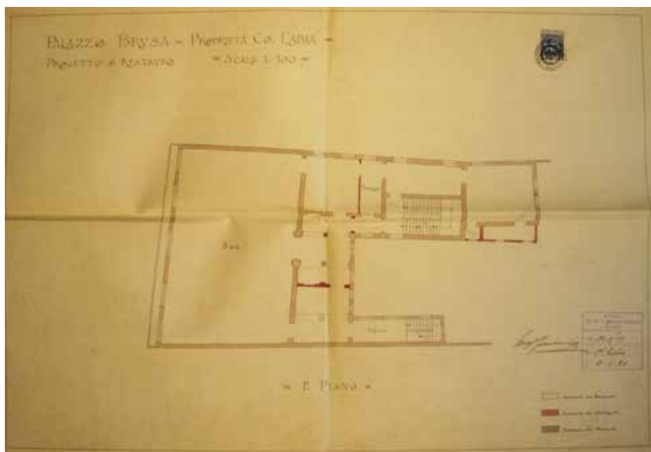
Figura 2. Pianta del primo piano
