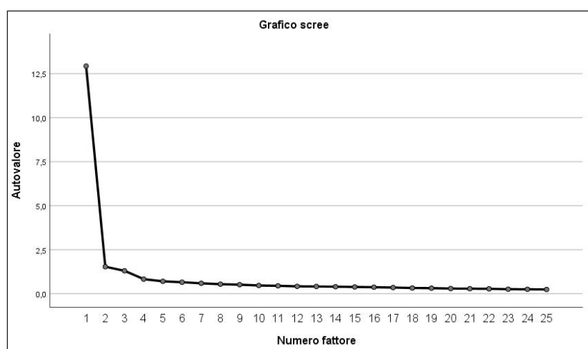
Figura 1: Scree-plot degli autovalori
