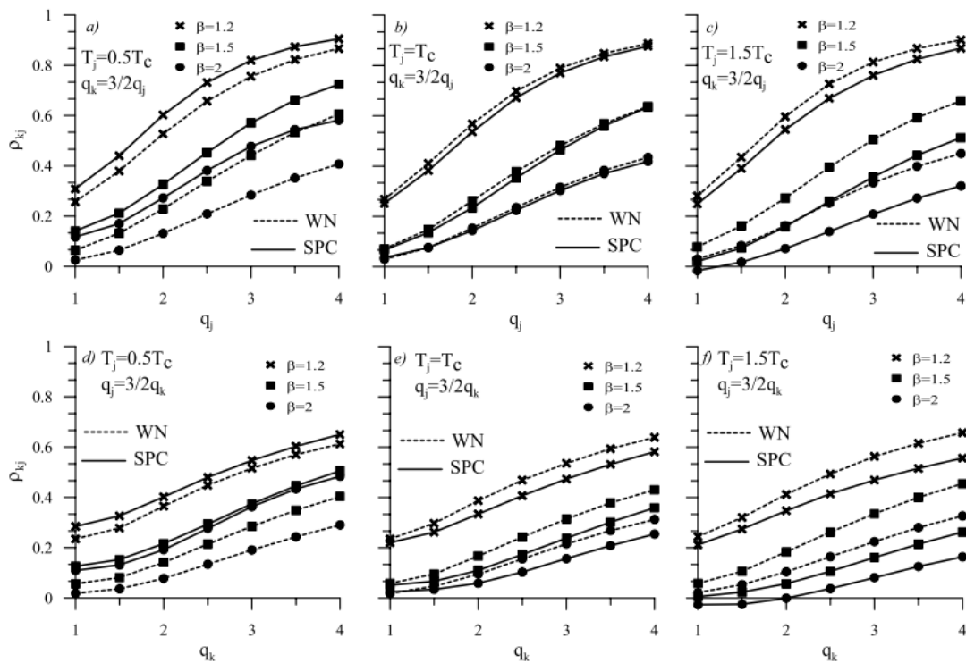
Figura.2 Influenza del fattore di struttura q sui coefficienti di correlazione non lineari, con rapporto di iniezione v_j=v_k=v=0.30 , coefficiente di smorzamento \zeta_i=\zeta_k=\zeta=0.05 ; a)-c) fattore di struttura q_k=3/2q_j ; d)-f) q_j=3/2q_k .
