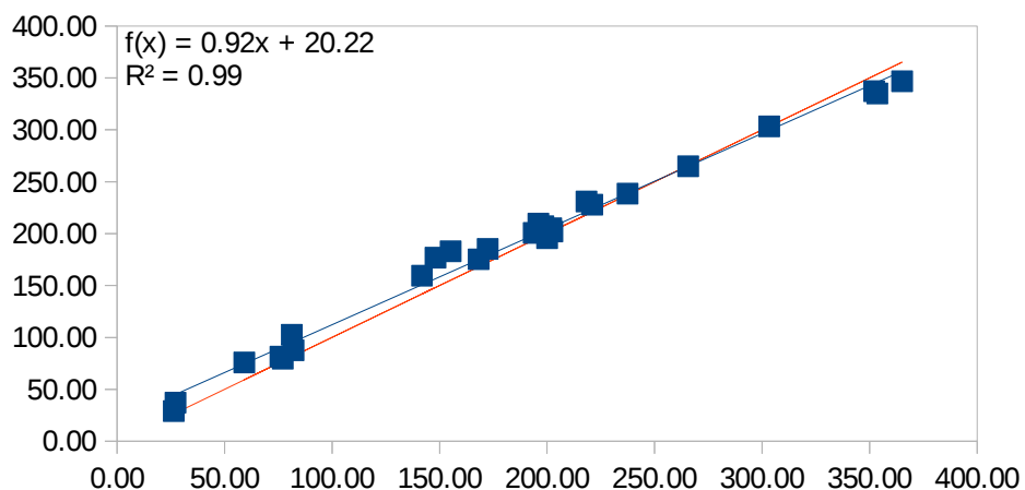
G09: B3LYP/Sadlej(Cd);6-31G+(d,p)//OP2
