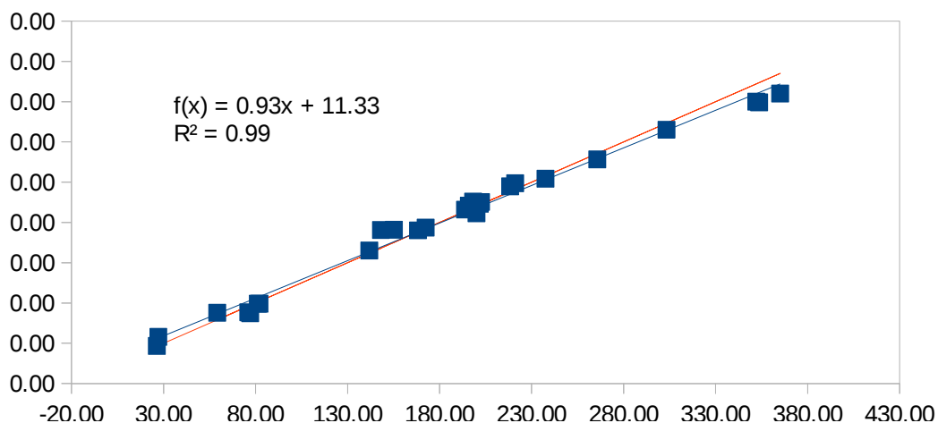
G09: B3PW91/Sadlej(Cd);6-31G(d,p)//OP2
