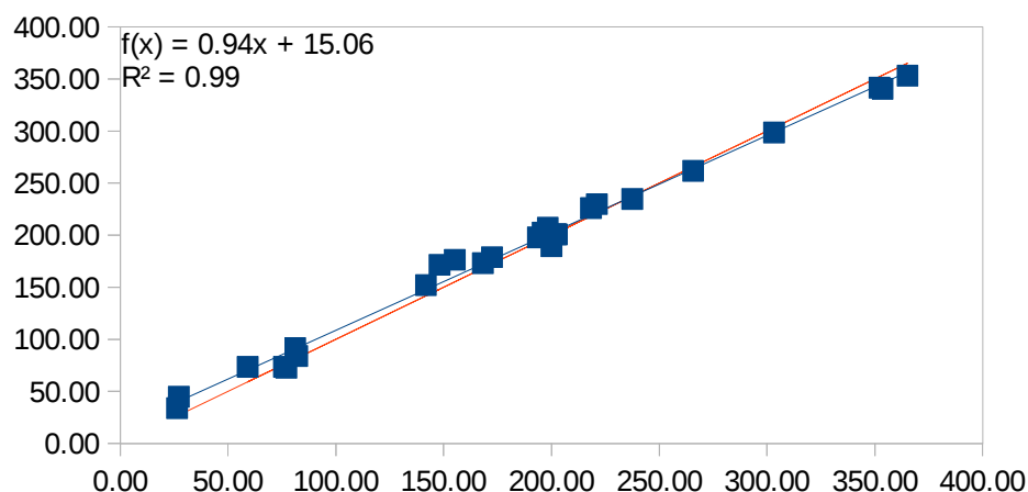
G09: B3LYP/Sadlej(Cd);6-31G(d)//OP2
