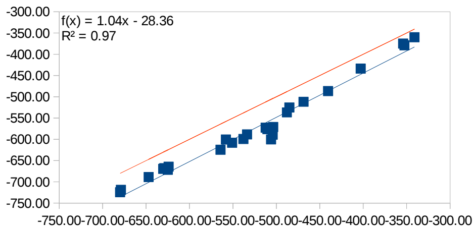
ADF: B3LYP/TZ2P//OP3
