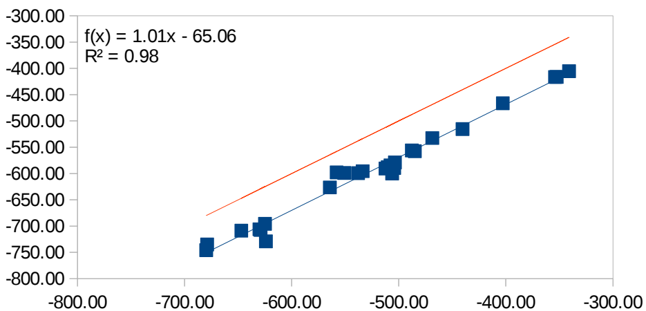
ADF: B3LY/DZP//OP2
