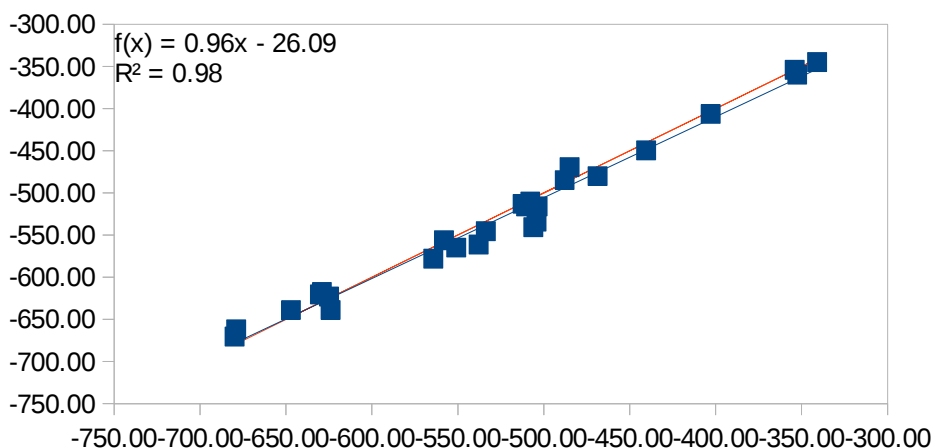
G09: B3LYP/Sadlej(Cd);6-31G(d)//OP3
