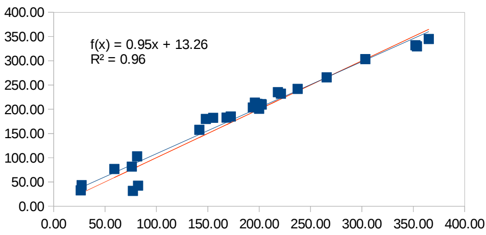
G09: B3PW91/Sadlej(Cd);6-31+G(d,p)//OP2
