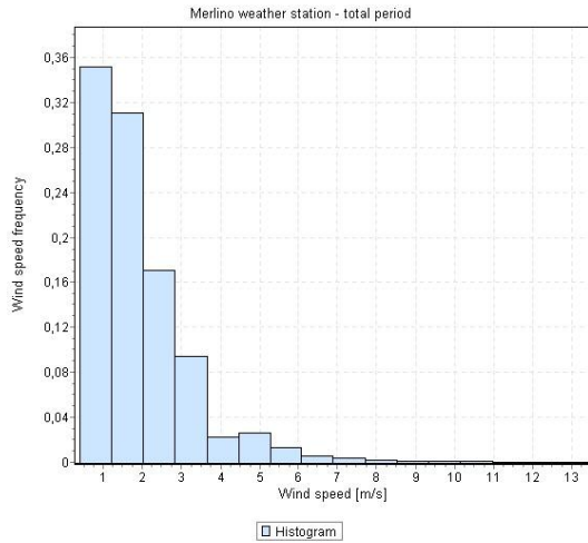
Figura 2: Istogramma della velocità del vento per la stazione meteorologica Merlino durante l'intero periodo di riferimento
