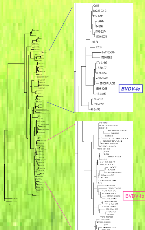
Figura 3. Albero filogenetico
