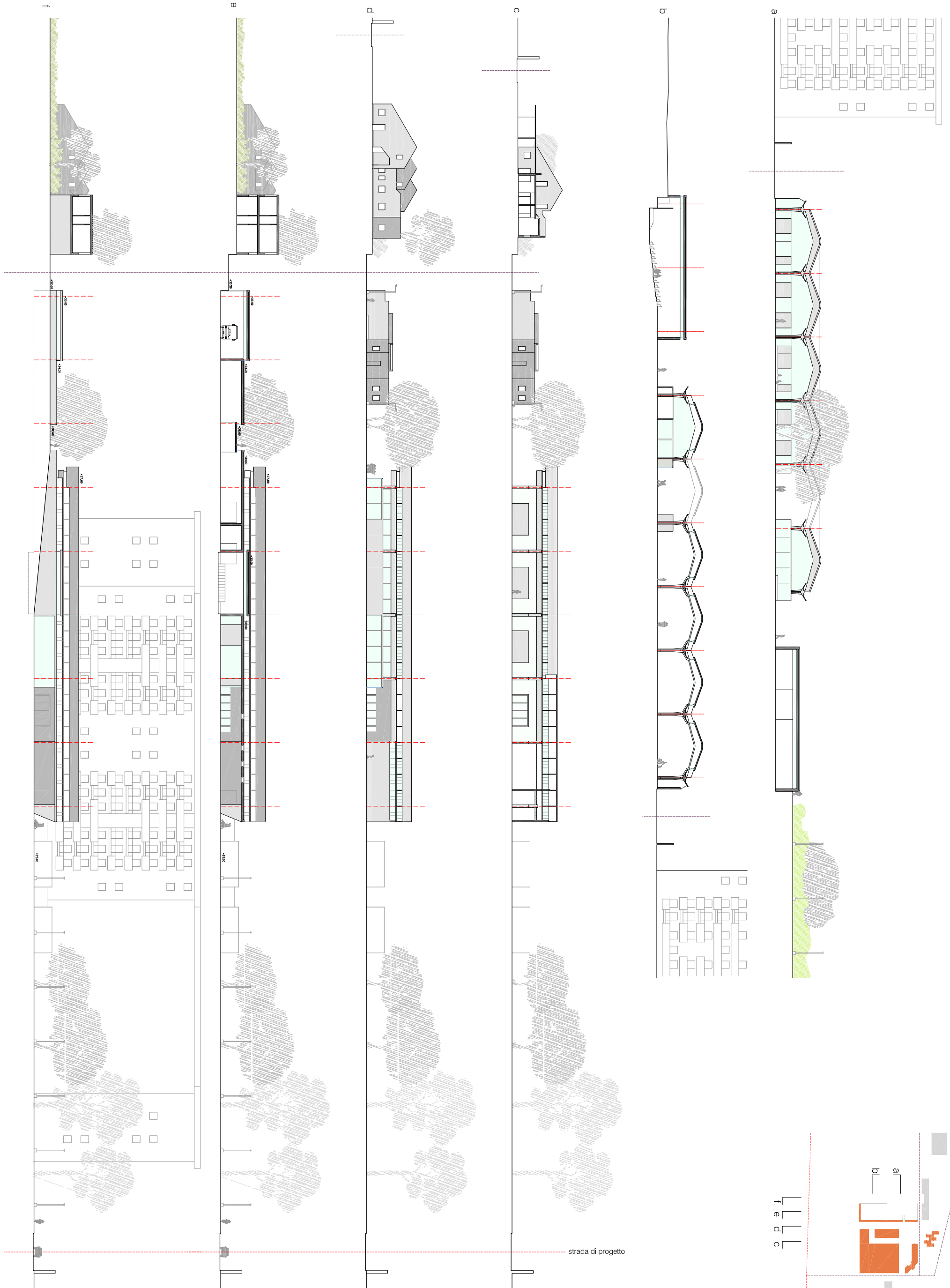
tav D3 - Sezioni generali
