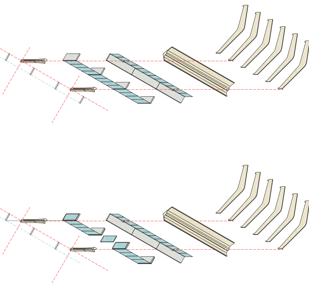
esplso assonometrico pilastro-trave-copertura
