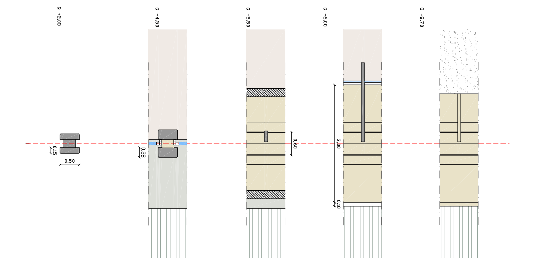
stratigrafia pilastro-trave-copertura
