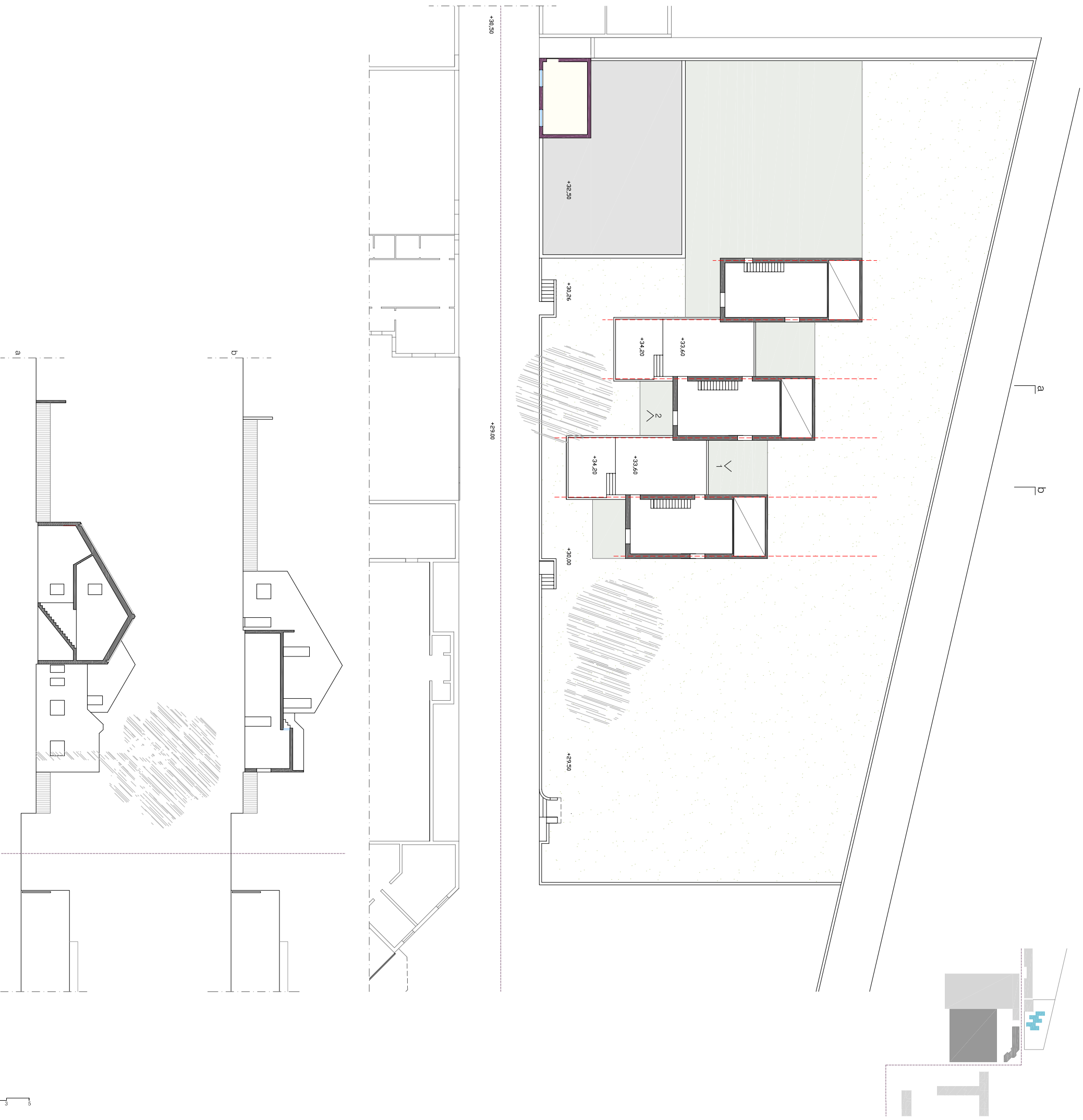
tav B5 - Residenze: pianta piano primo e sezioni
