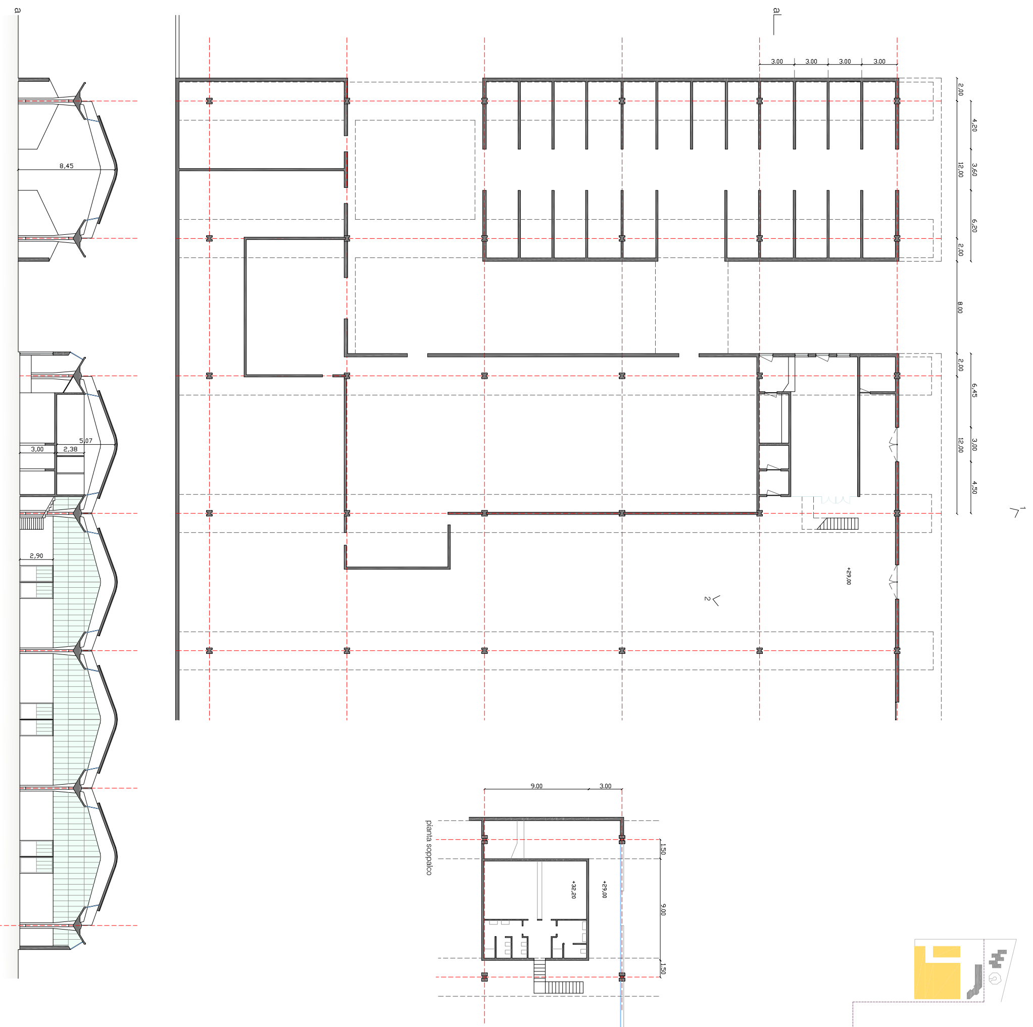
tav A7 - Fabbrica: Pianta e sezioni
