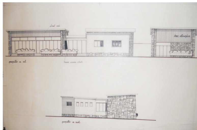
1949-57 QUARTIERE MALASPINA-NOTARBARTOLO Progetto di centro assistenziale, gruppo di negozi e bar Archivio Salvatore Caronia Roberti
