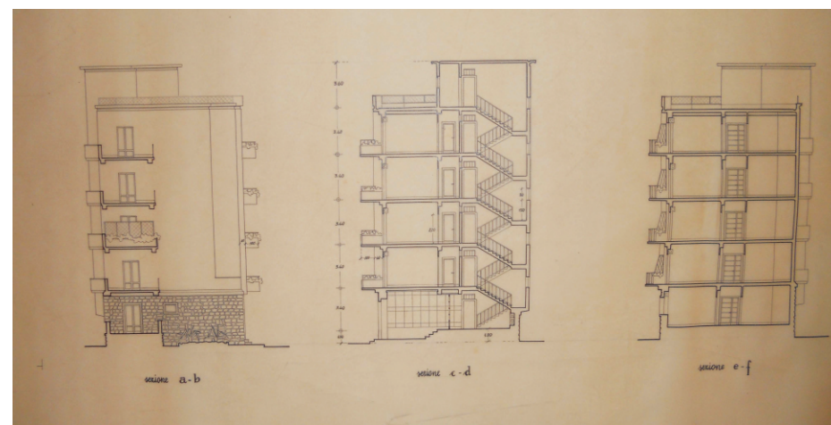
1949-57 QUARTIERE MALASPINA NOTARBARTOLO Edificio d1 - prospetti e sezioni Archivio Salvatore Caronia Roberti
