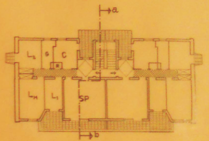
pianta del piano tipo
