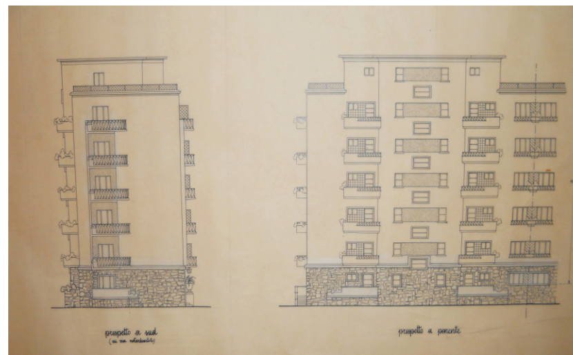
1949-57 QUARTIERE MALASPINA NOTARBARTOLO Edificio d - Pianta e prospetti Archivio Salvatore Caronia Roberti
