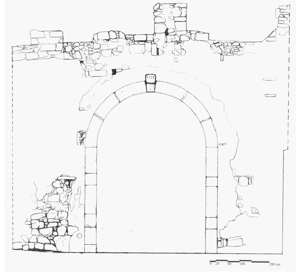
Prospetto esterno
