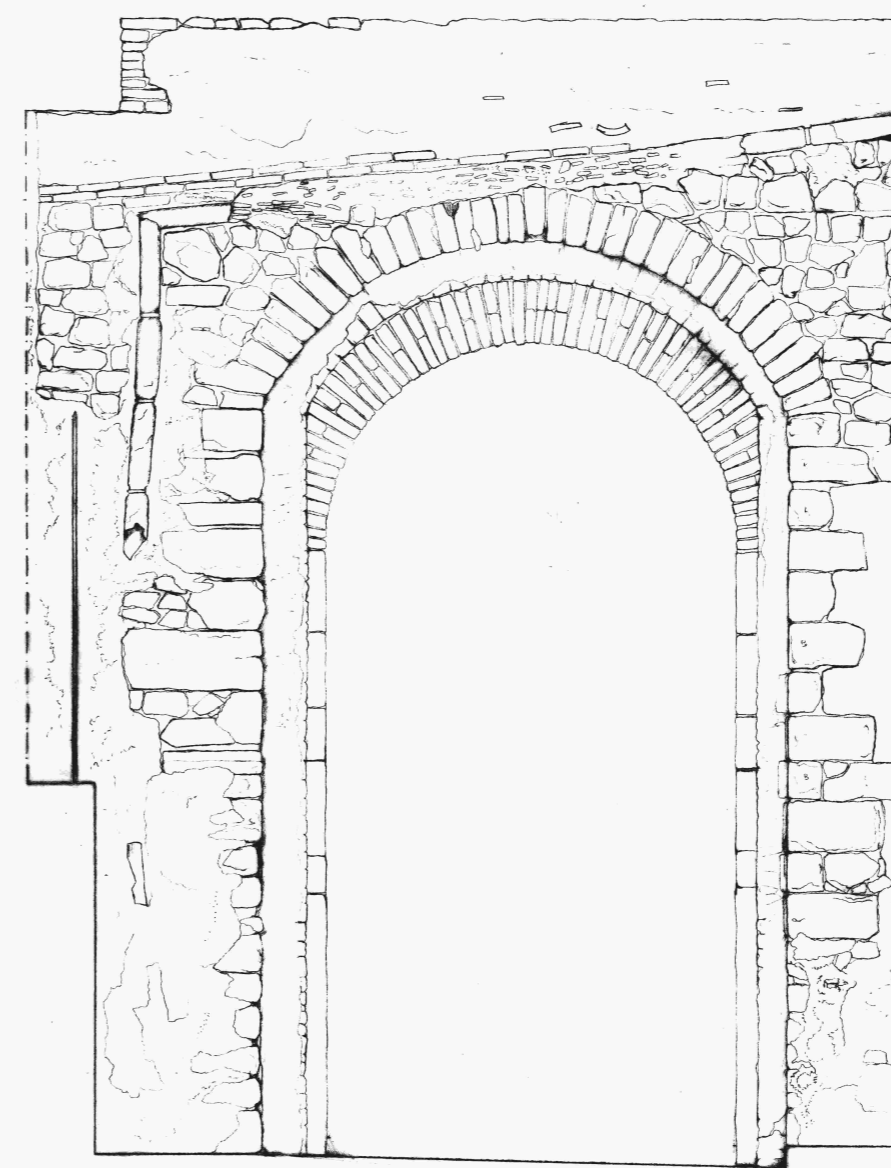
Prospetto esterno
