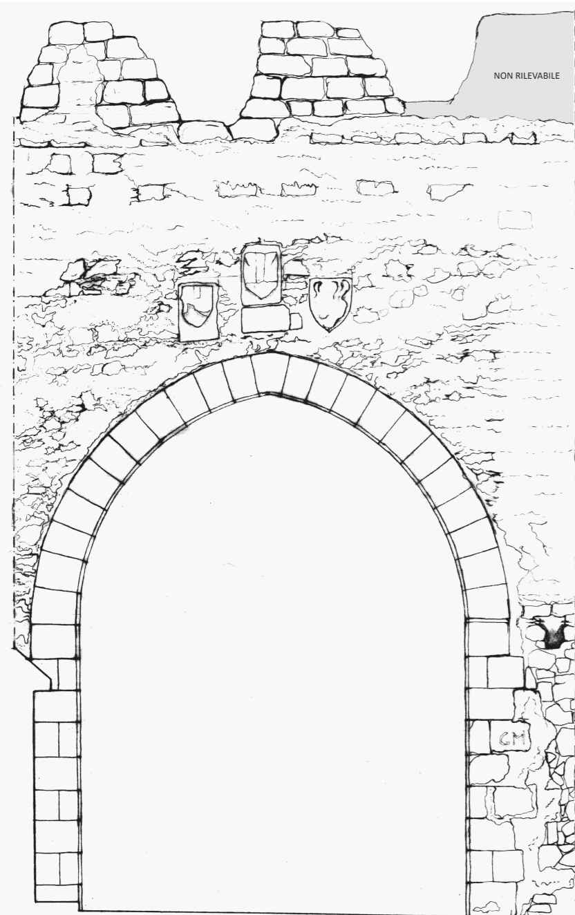
Prospetto interno
