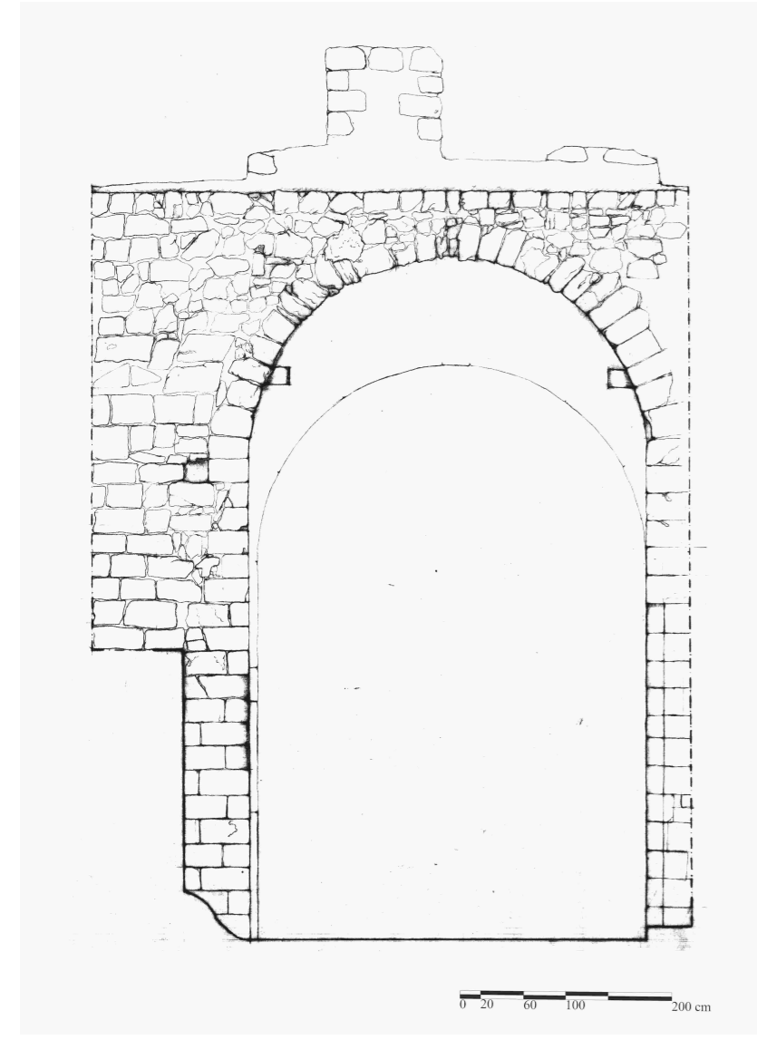
Prospetto interno
