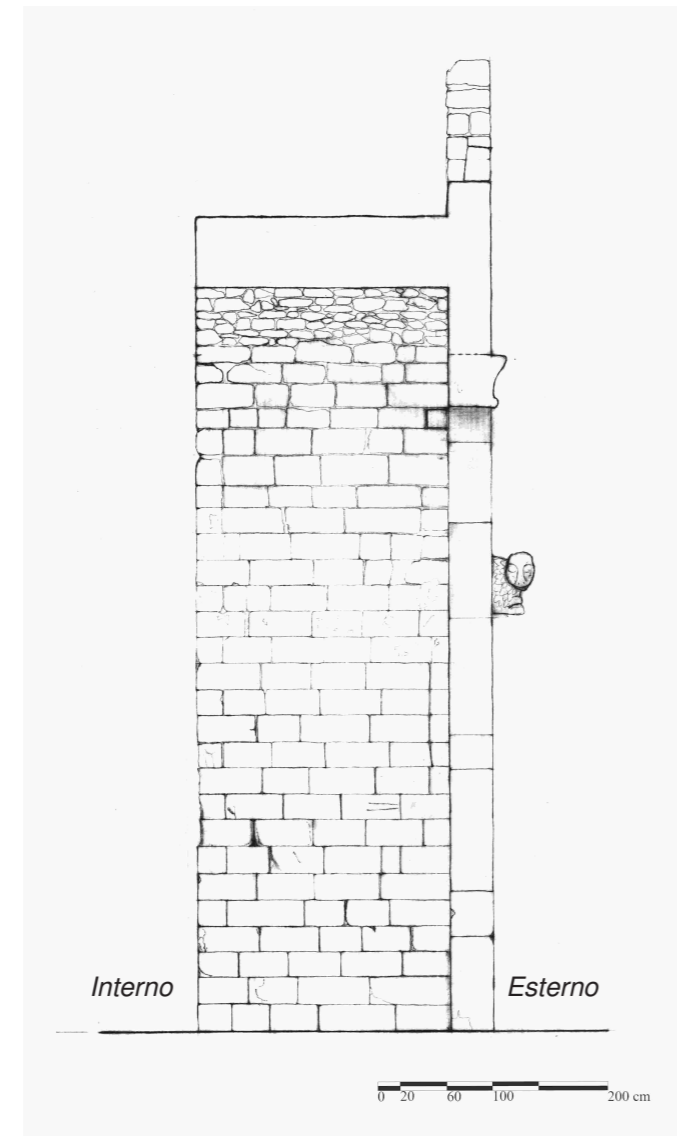
Sezione
