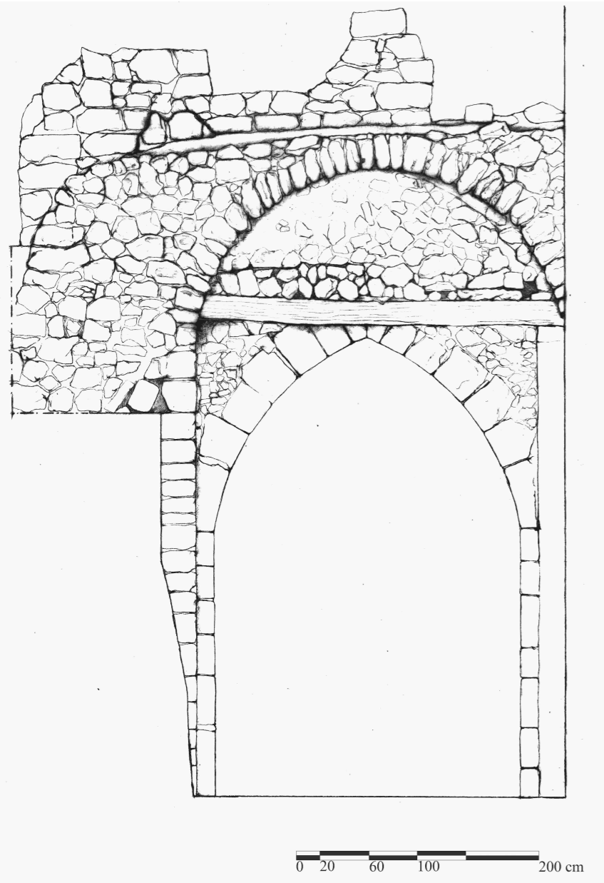
Prospetto interno
