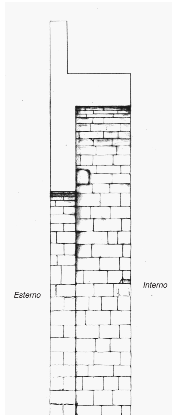
Sezione
