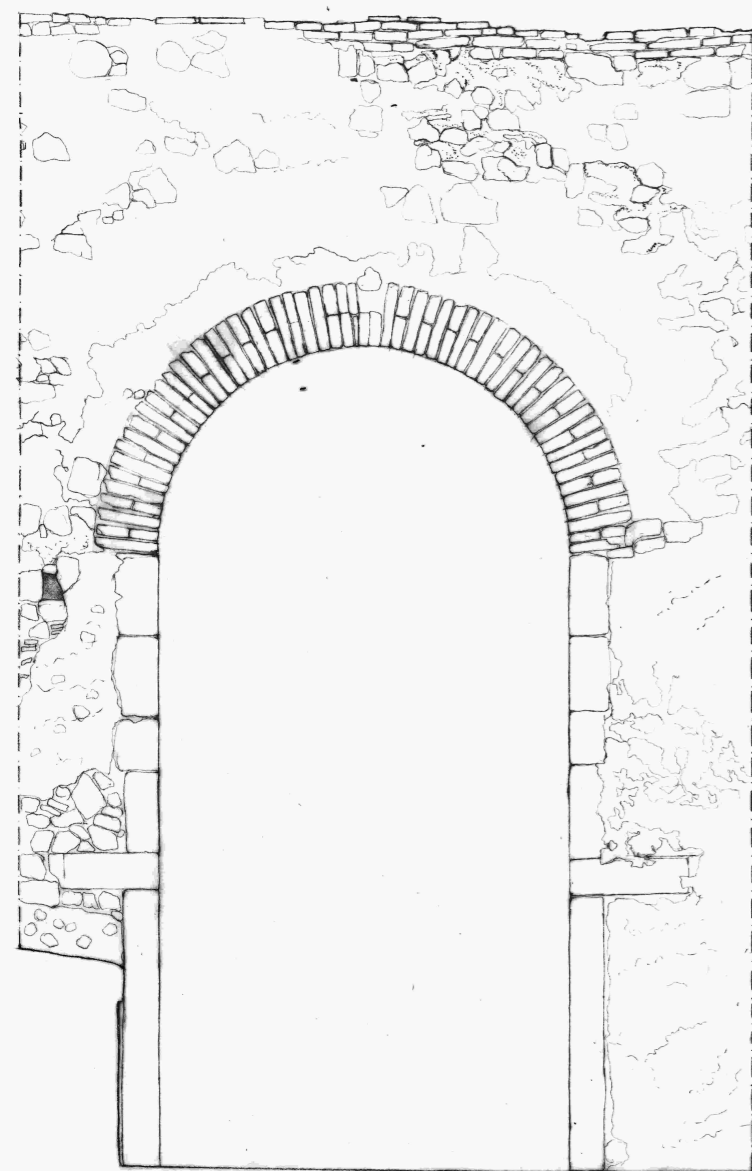
Prospetto interno
