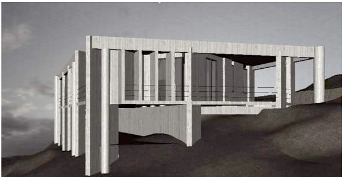
TAV. XVII – CASA TIAR A PALERMO, 1976-1977 (restituzioni tridimensionali a cura dell'Arch. Claudia Granata, Bagheria 2013)
