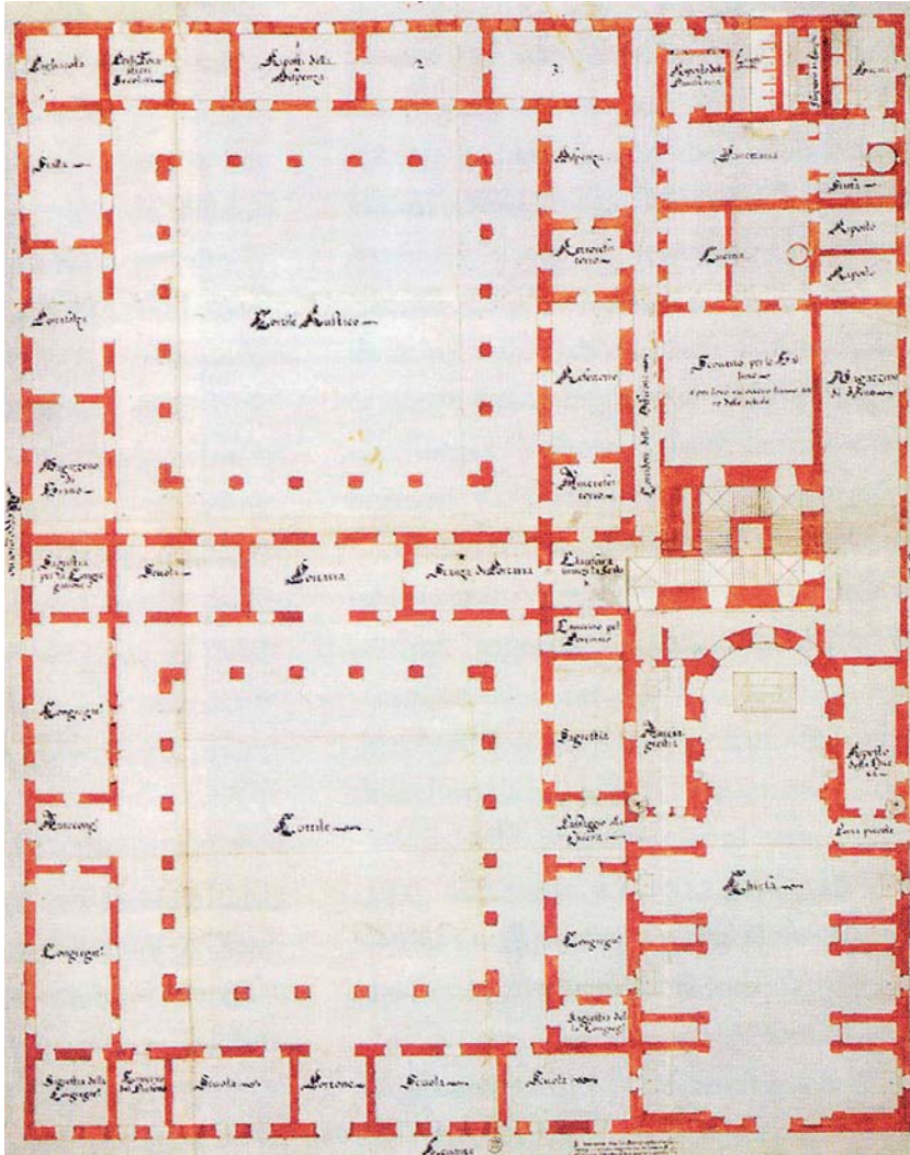
Fig. 16. Modica. Planimetria del complesso gesuitico (B.N.P., Hd-4b, 1; V. R. n. 197). Foto: Proyecto Corpus de arquitectura jesuítica.
