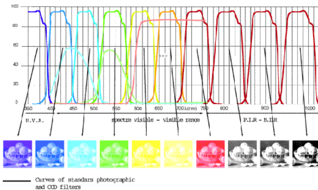
Fig. 2 Curve spettrali e filtri
