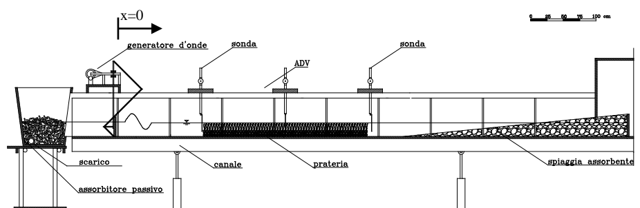
Figura 2. Vista laterale del canale del Laboratorio di Idraulica dell'Università degli Studi di Catania.
