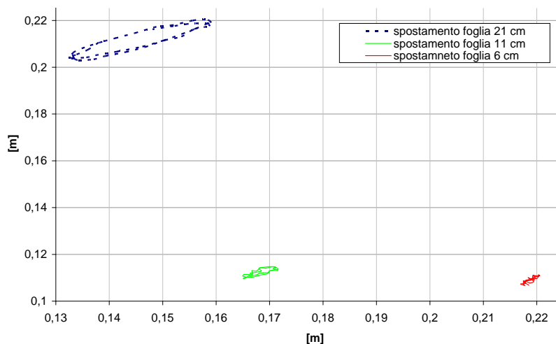
Figura 7. Spostamenti degli apici delle foglie di una singola pianta artificiale di Posidonia Oceanica .
