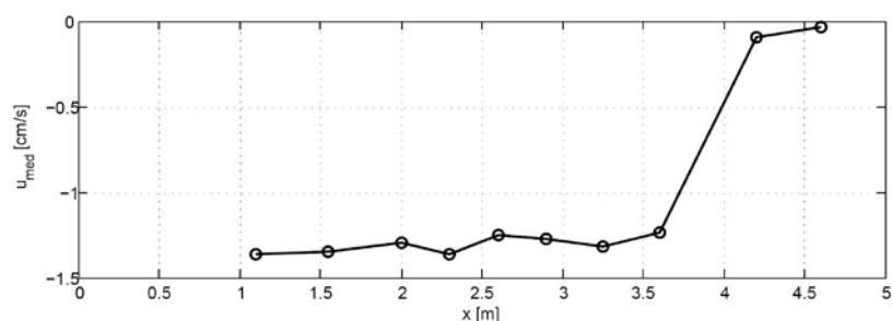
Figura 3. Distribuzione della velocità media lungo x misurata ad una profondità di circa 13 cm rispetto al livello di quiete. L'onda in ingresso ha: H = 4,5 cm ; T = 0,74 s.
