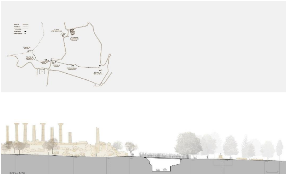
Fig.4. Sezione del ponte e il tempio di Eracle, Cottone+Indelicato (2012-2015).
