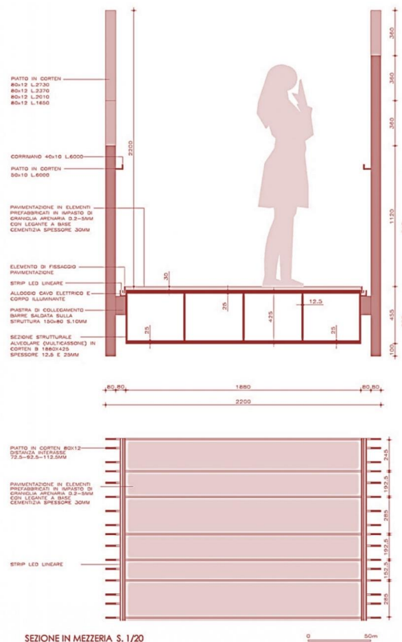
Fig.4. Sezione del ponte per il parco archeologico di Agrigento, Cottone+Indelicato (2012-2015).
