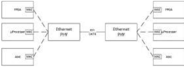
Fig. 3.35. Ethernet subsystem.
