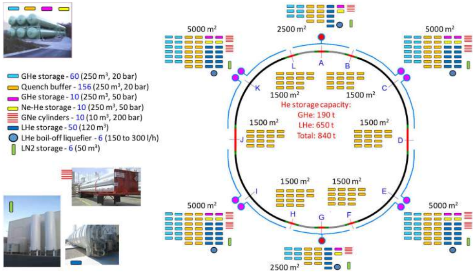
Fig. 5.19. Cryogen storage.
