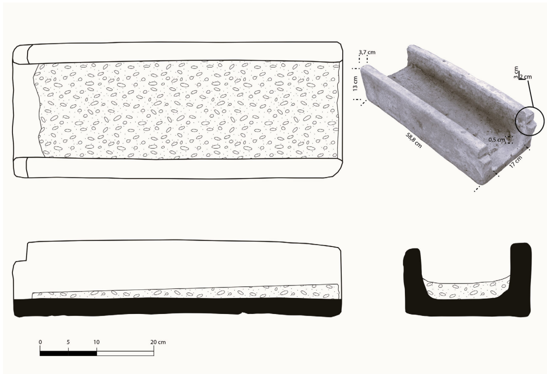
Fig. 57 Segesta, depositi del Parco Archeologico, inv. 17165. Elemento (I) della canaletta a cassetta, foto e restituzione grafica.
