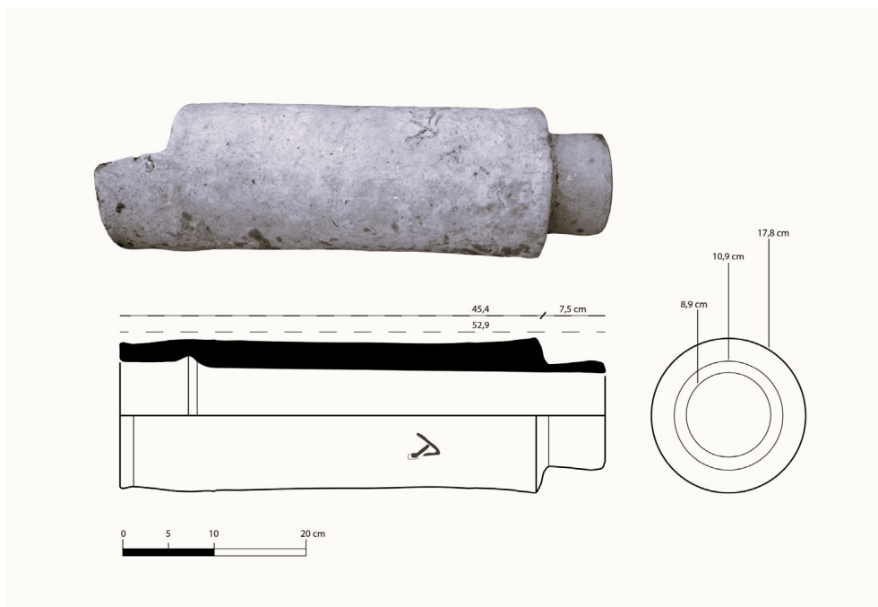
Fig. 55 Segesta, depositi del Parco Archeologico, inv. SG 17163. Tubulo V della canaletta cilindrica, foto e restituzione grafica.
