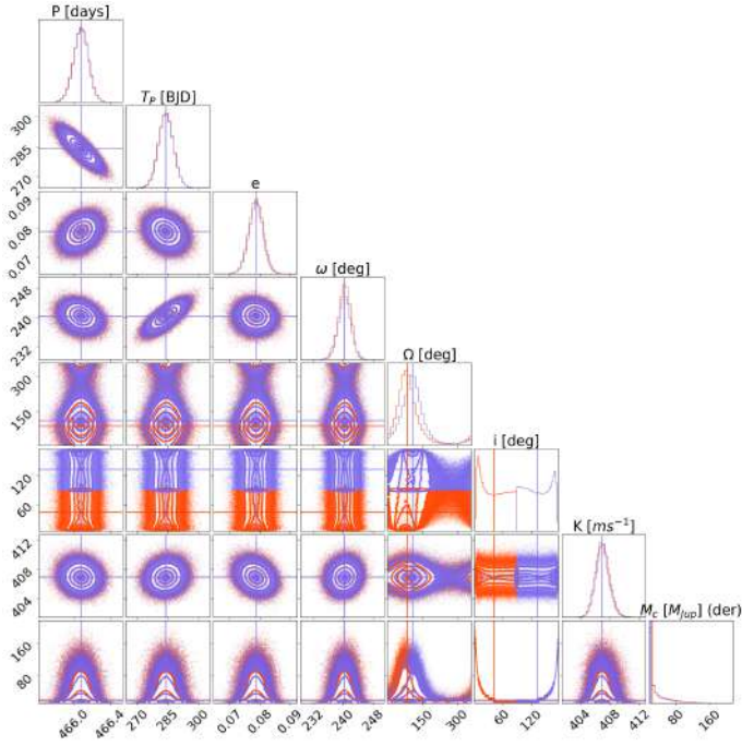
Fig. B.6. Posterior distributions of HD 16760 system.
