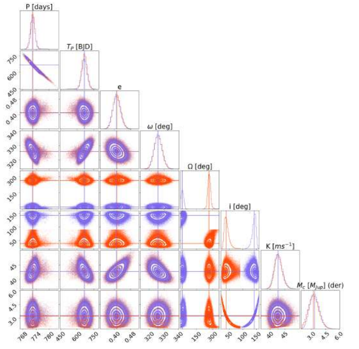
Fig. B.4. Posterior distributions of HD 5388 system.
