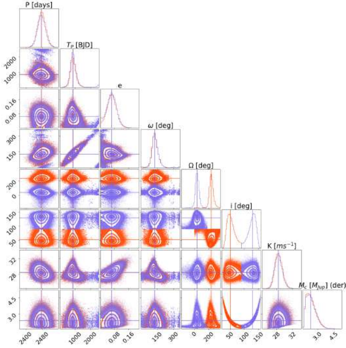
Fig. B.5. Posterior distributions of HD 6718 system.
