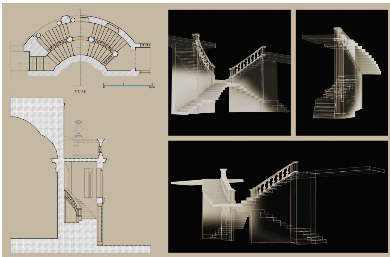
Fig. 3. Ridisegno e lettura grafica: piante, sezione e ricostruzione tridimensionale del particolare della scala del progetto di Paolo Labisi.
