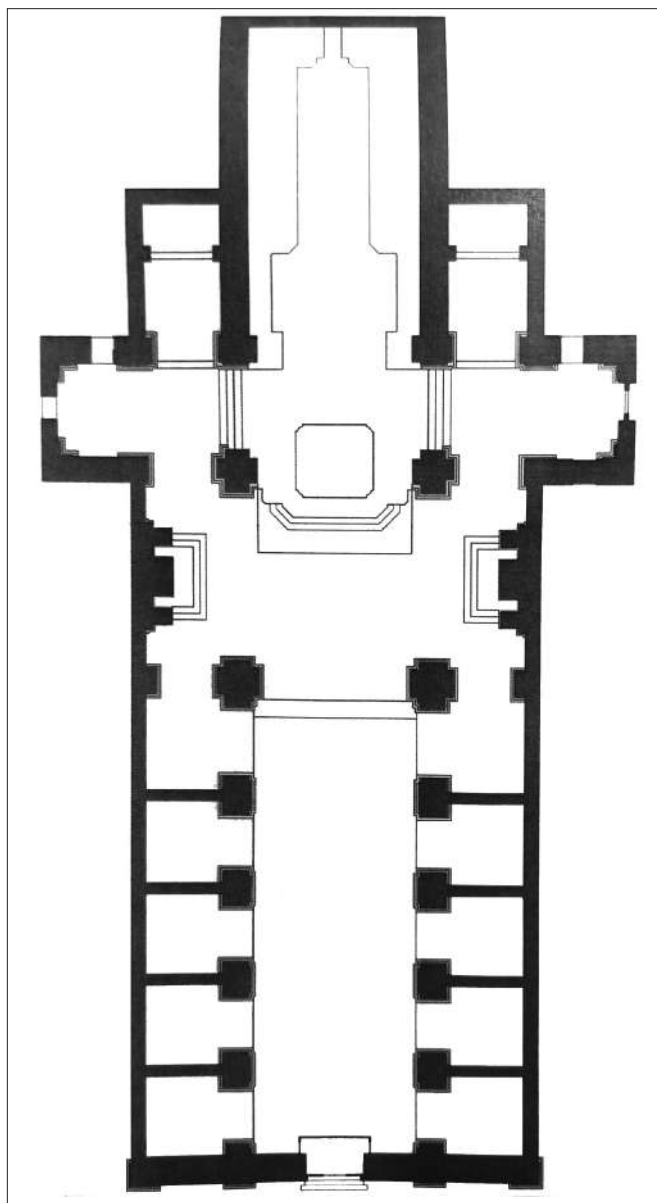
Fig. 1. San Martino delle Scale (Palermo), chiesa abbaziale; pianta (elaborazione grafica di Simona Silvoia).
