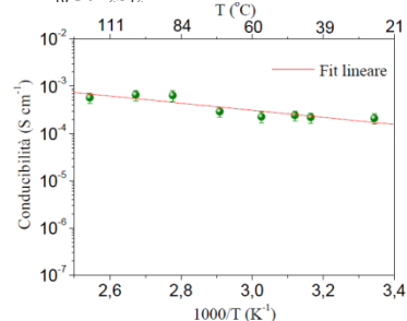
Figura 1: Arrhenius plot dell'elettrolita \text{Li}_{10}\text{GeP}_2\text{S}_{12}
