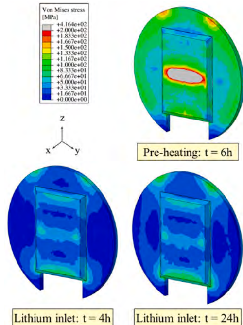
Fig. 19. BPL Von Mises stress field - view1.
