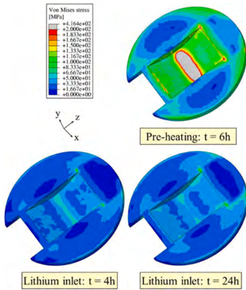
Fig. 20. BPL Von Mises stress field - view2.
