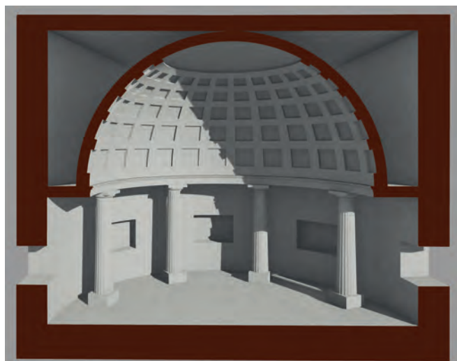
Fig. 3. Ricostruzione prospettica del "parlatoio" del monastero di Santa Lucia a Siracusa (elaborazione grafica a cura dell'autrice).
