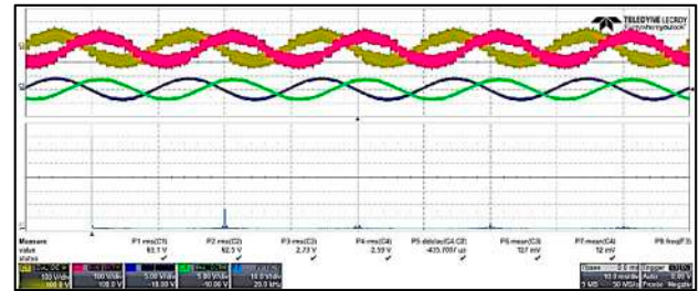
(d) SFOPD: M = 0.9 - f_{sw} = 40 kHz
